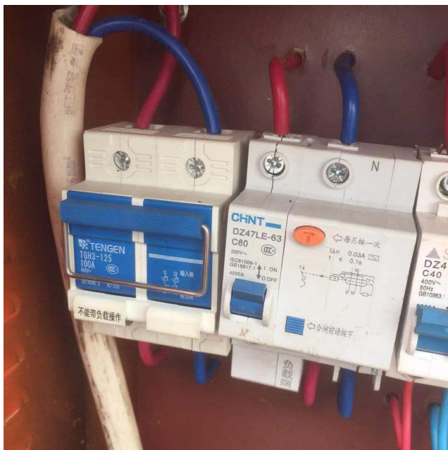
项目部总开漏保不动作未更换
