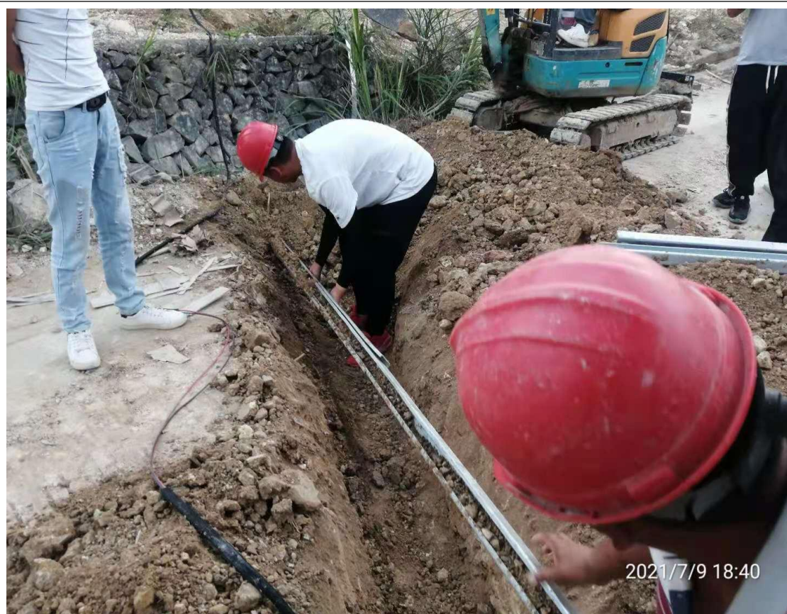
过路电缆线未按设计、规范要求施工
