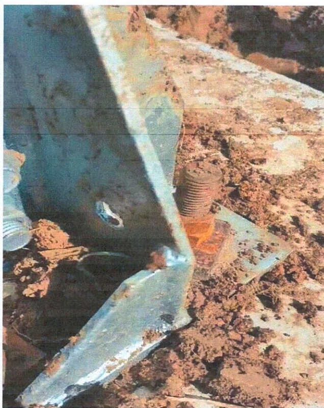
相片四：地脚螺栓未拧紧
