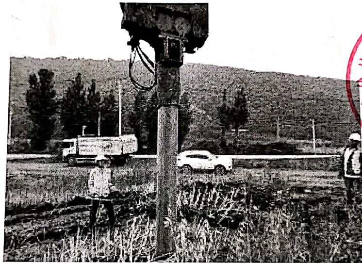
桩基垂直度调整
