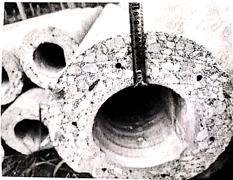
壁厚不符合要求的管桩已更换
