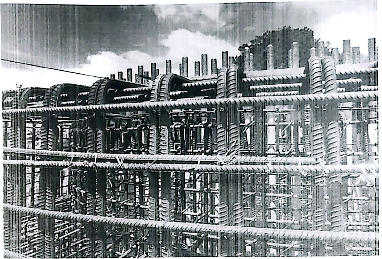
6#风机基础钢筋
