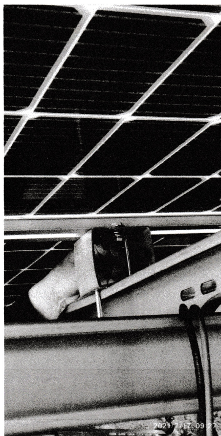
组件中间压块螺栓未紧固
