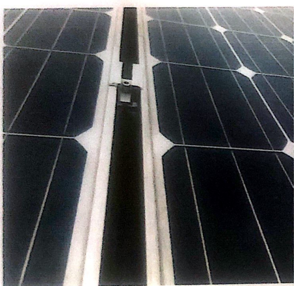
组件压块存在缝隙
