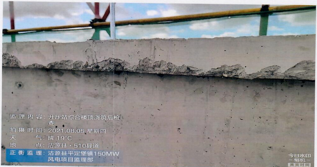
图 1：拆模过程或其他问题没有注意成品保护
