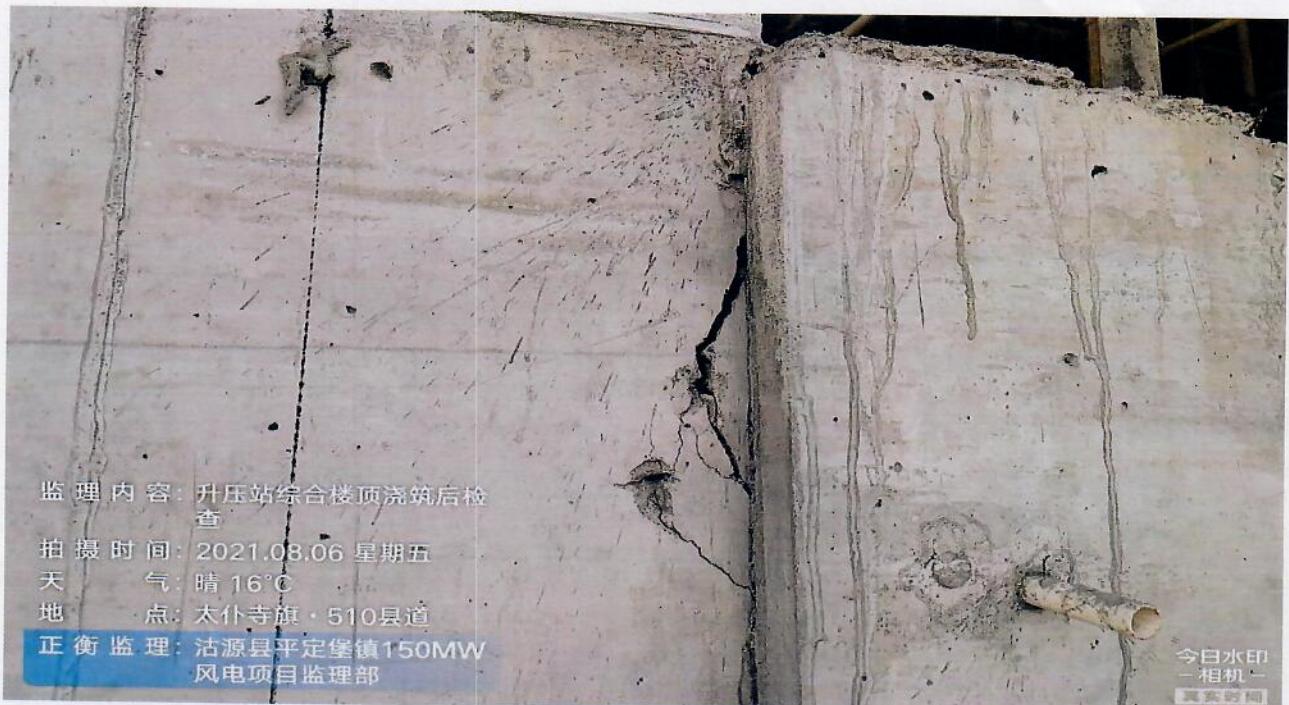
图 2：漏振或振捣不到位。
