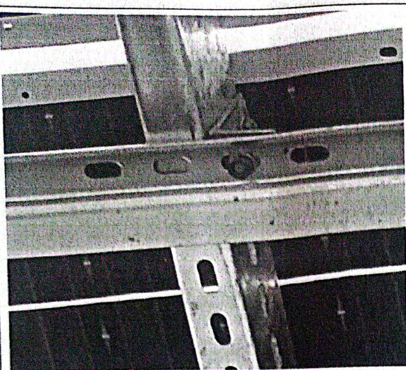
斜梁与檩条处未安装螺栓
