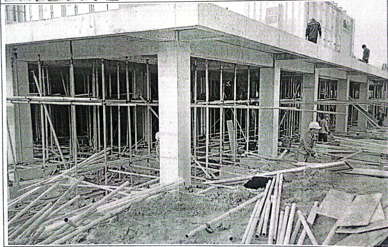
升压站基础平台已开始拆模
