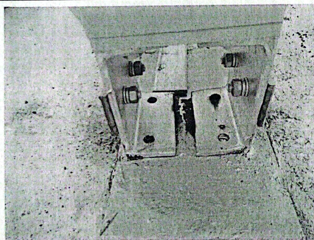
SVG 电抗器围栏焊接处焊渣未清理
