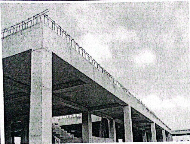
综合楼二层及平台大门处未设置临边防护
