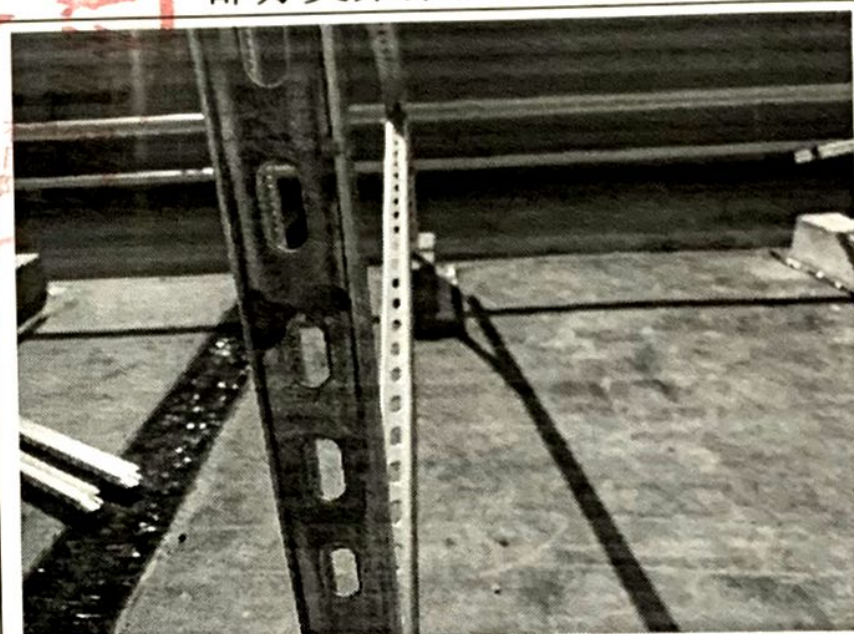
个别支架立柱锈蚀
