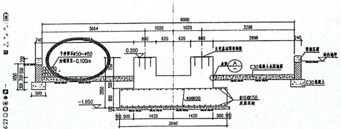
1-1 剖面图 1:50
