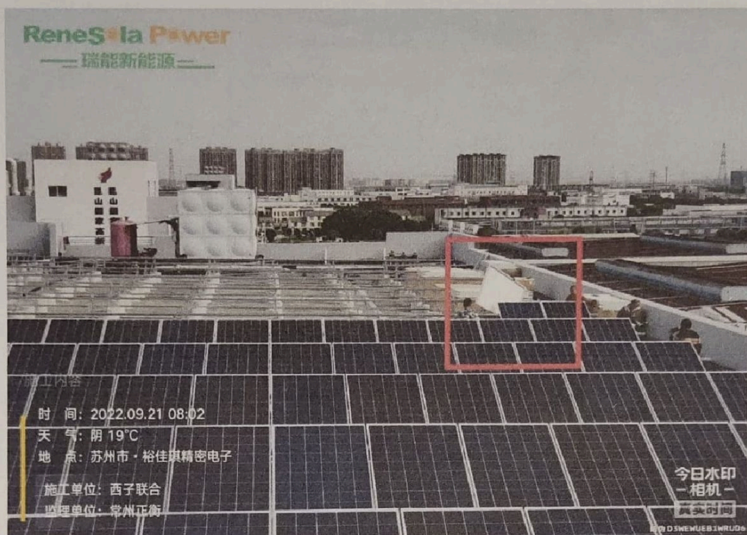
2 号楼单人搬运组件
