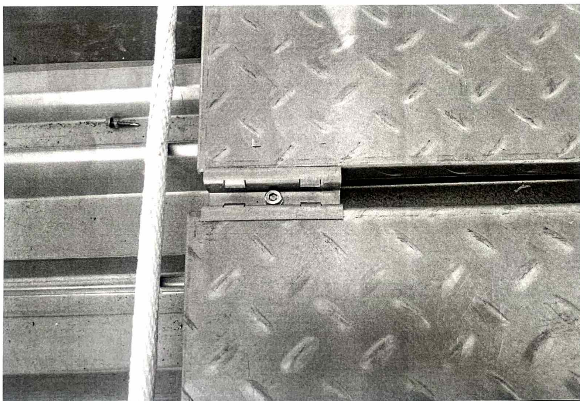
过道板压块未压接到位
