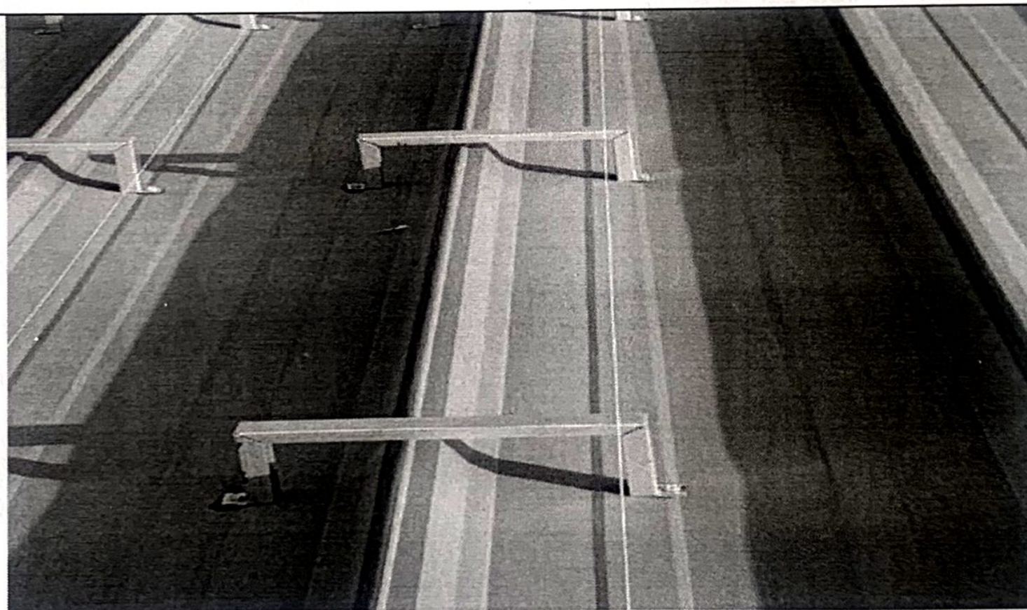
马凳安装不顺直
