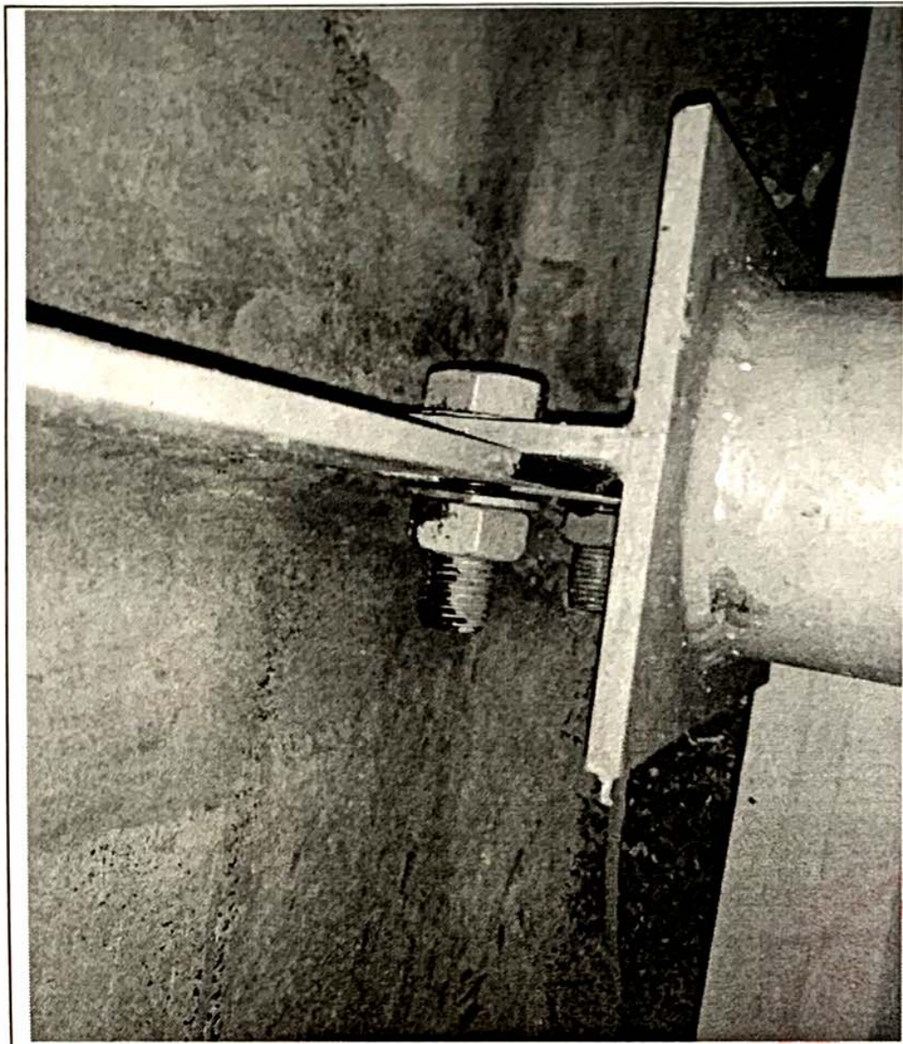
系杆紧固件螺栓未紧固到位
