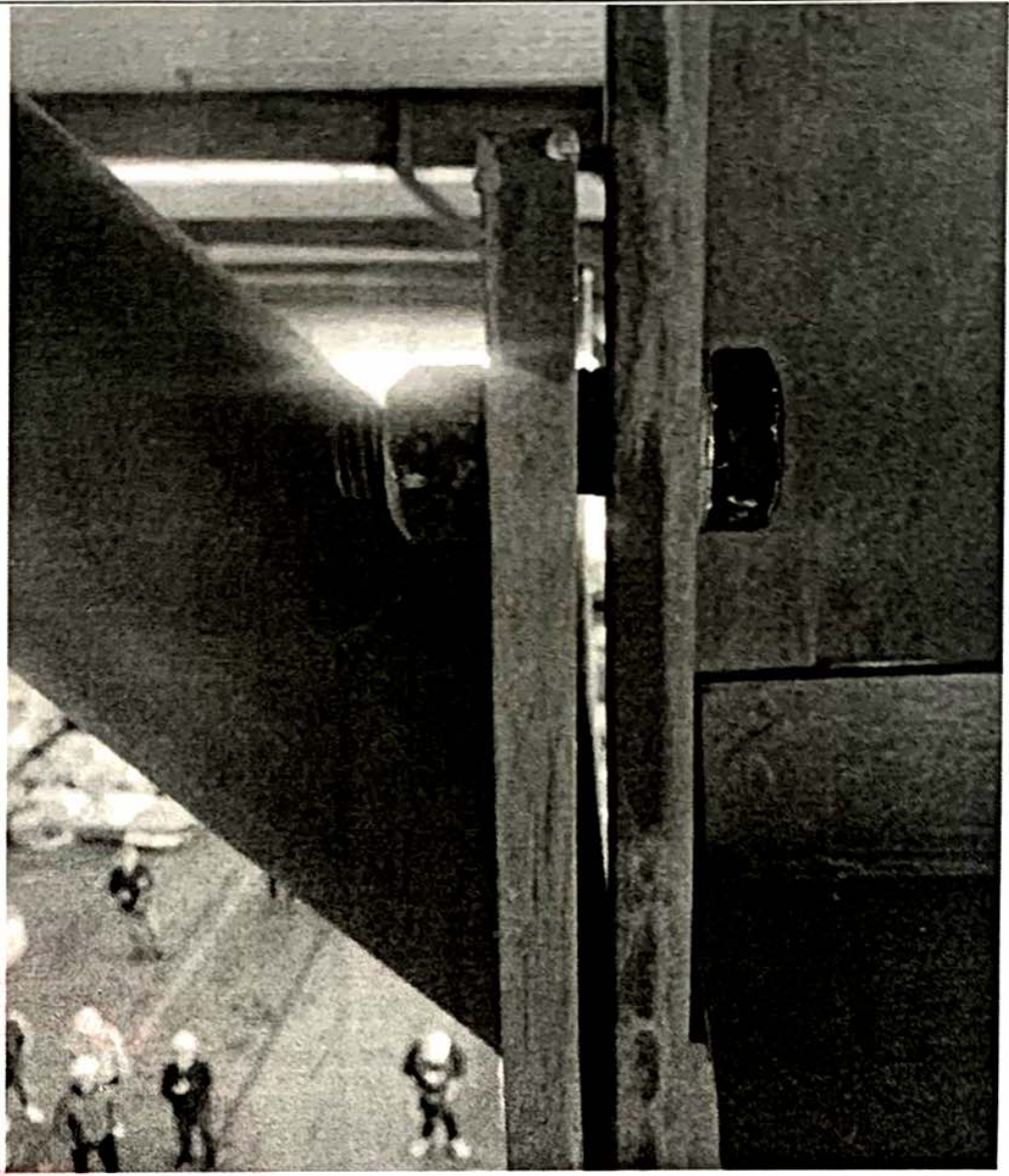
撑杆底板与横梁缝隙较大
