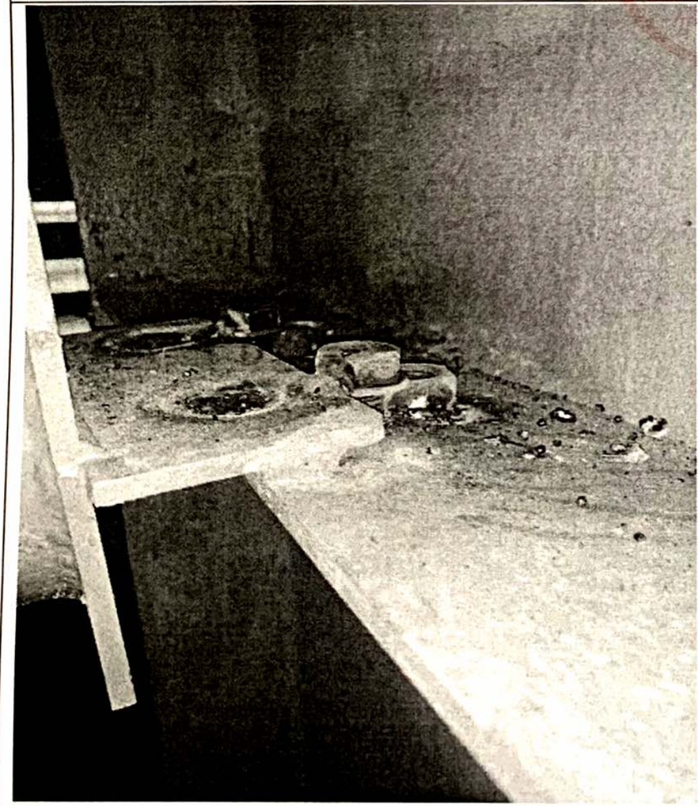
较短系杆焊接面积较少
