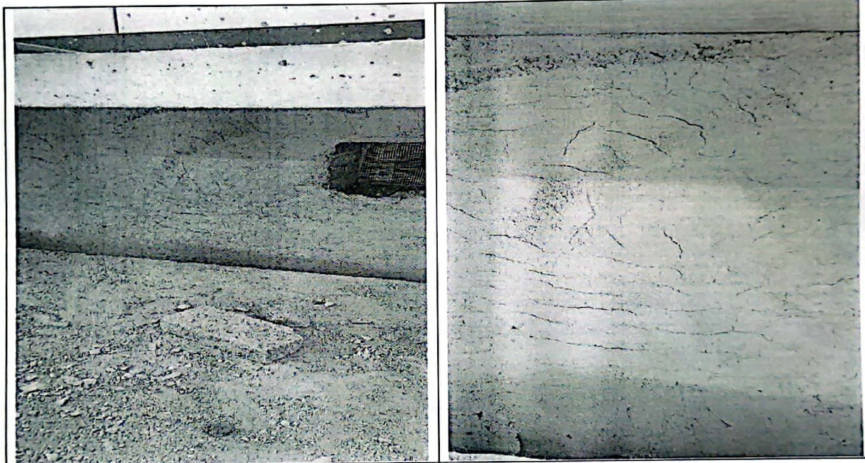
未使用防裂网，有较多裂缝
