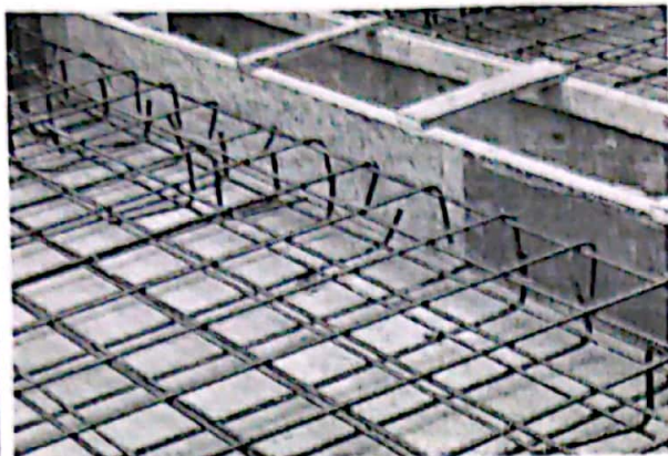
钢筋留置已按要求整改
