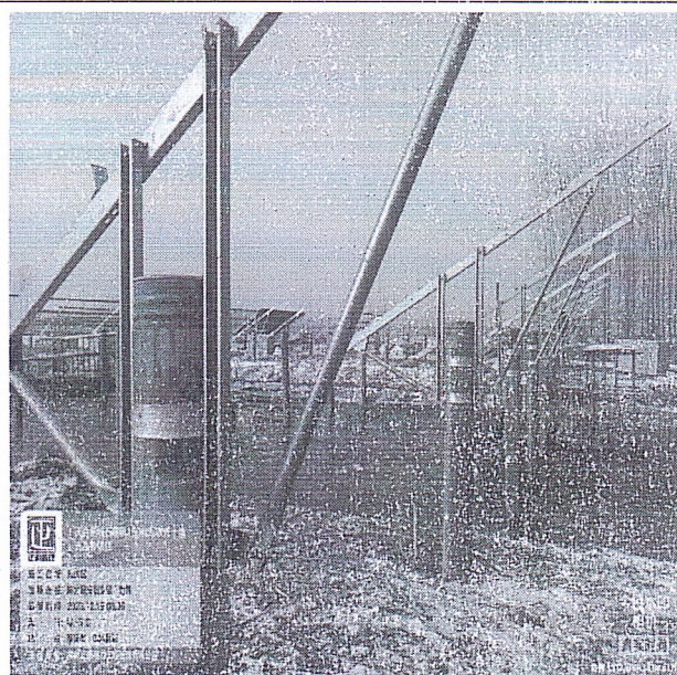
桩头未做防腐处理
