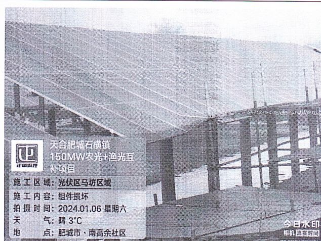
二期马坊组件受损
