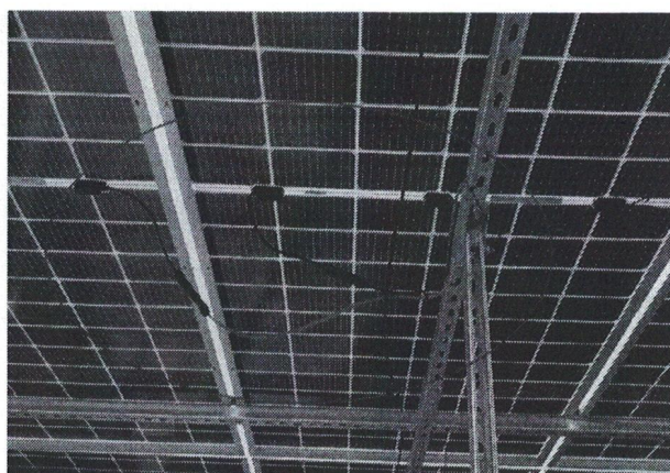
光伏电缆凌乱未绑扎固定
