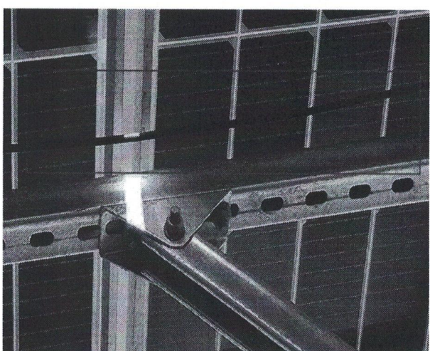
光伏电缆未穿管
