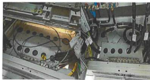
盘柜内垃圾未清理，无防火封堵
