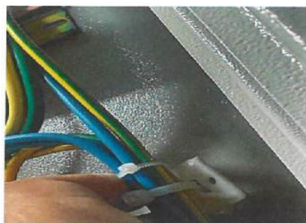
8. 缆固定节点脱落
