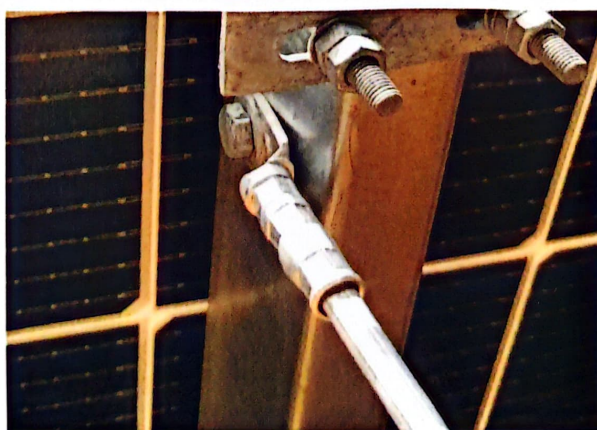
9. 组串接地安装不规范
