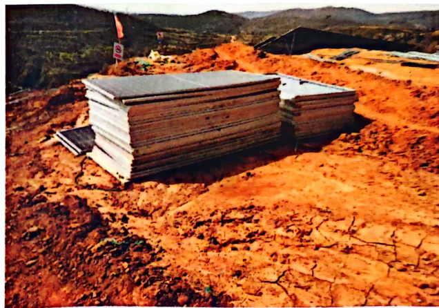
6. 斜梁弯曲导致组件波浪形
