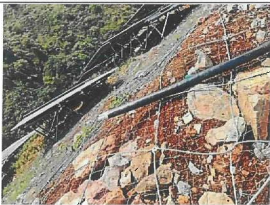
图 4：电缆终端未做保护
