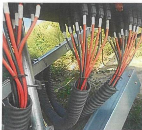
逆变器电缆防火封堵不符合要求
