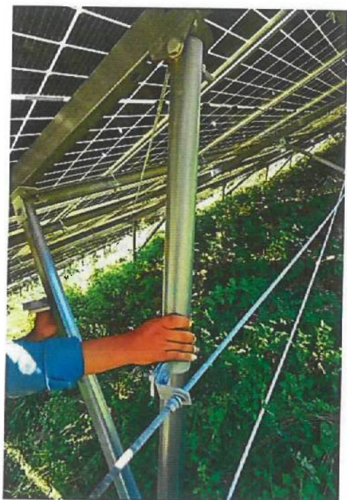
17-10-17管拉杆需要向上调整。
