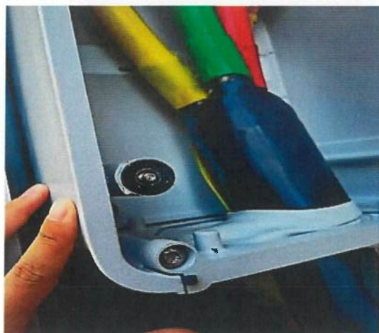
0703逆变器内部防火封堵未做。
