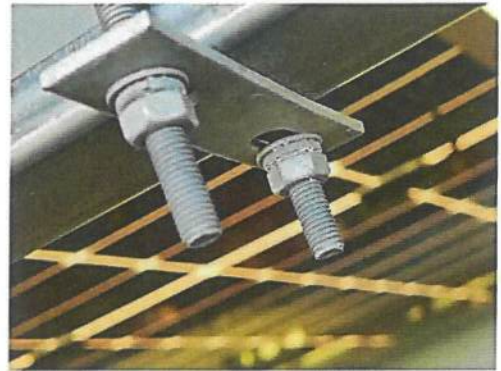
070313压块未做双螺母。多数，属于质量通病
