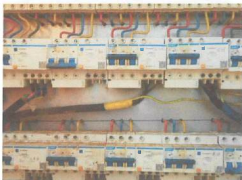
安装箱门跨接线，拆除一闸多用的电缆线
