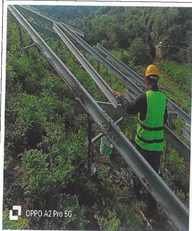
標条拆除調整
