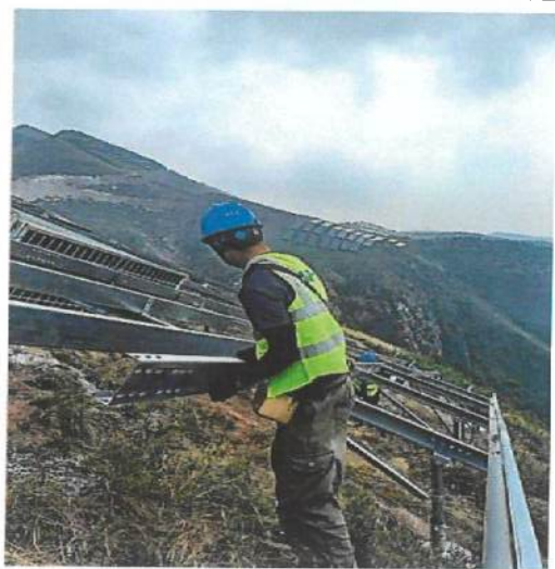
拆除装错檩条
