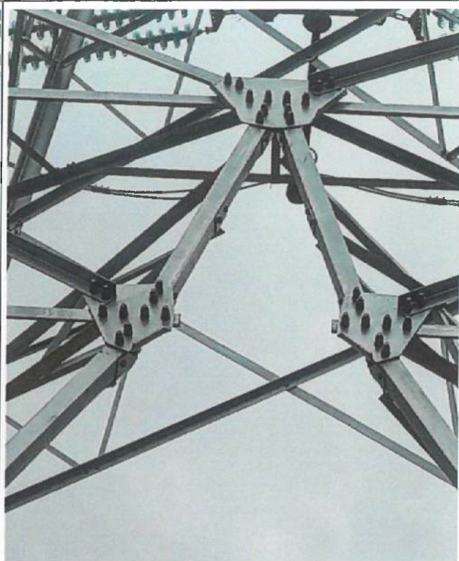
2、送出 G14 塔基缺少防盗帽且未拧紧
