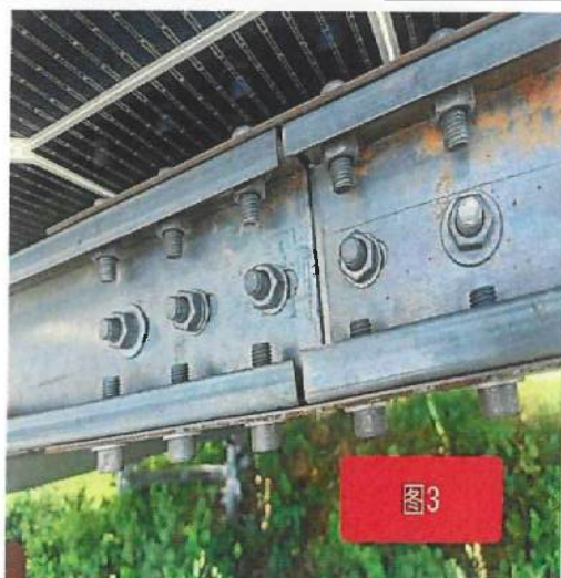
没有平垫弹垫已消缺
