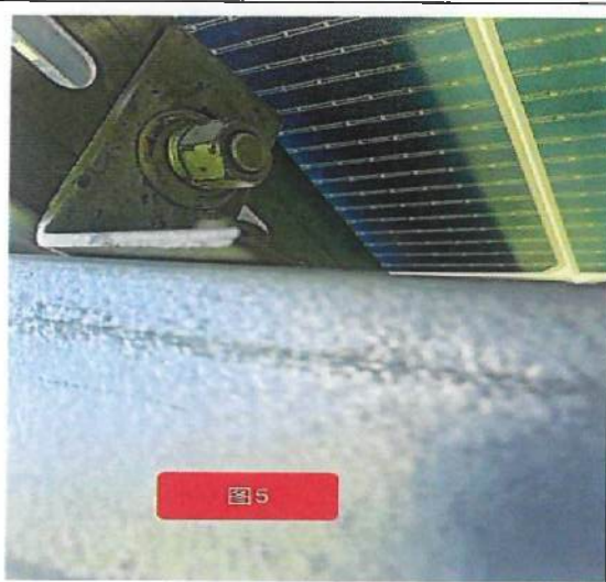
没有平垫弹垫已消缺
