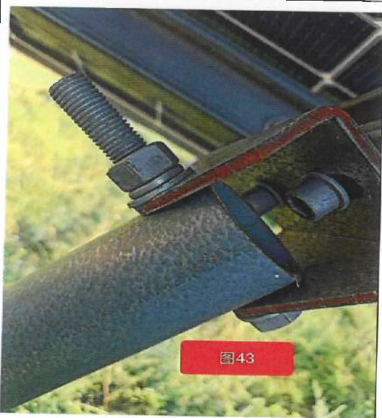
立柱螺丝未紧已整改
