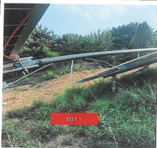
PE 管太短已整改
