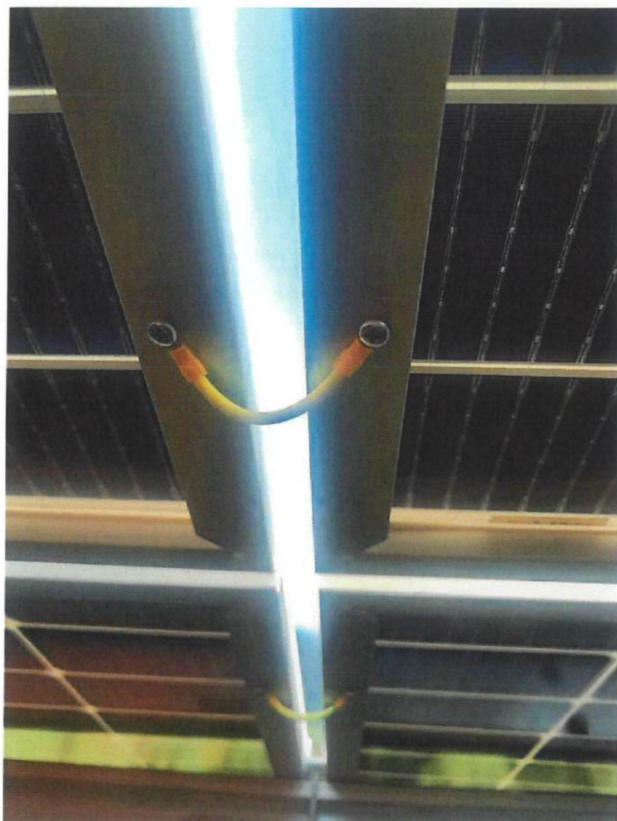
黄绿线连接
