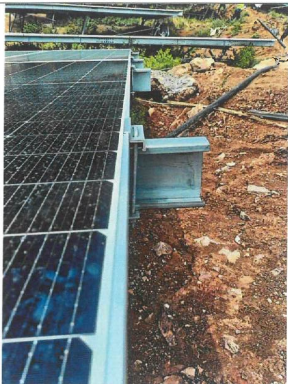
標条側边长度预留调整，保证边压受力
