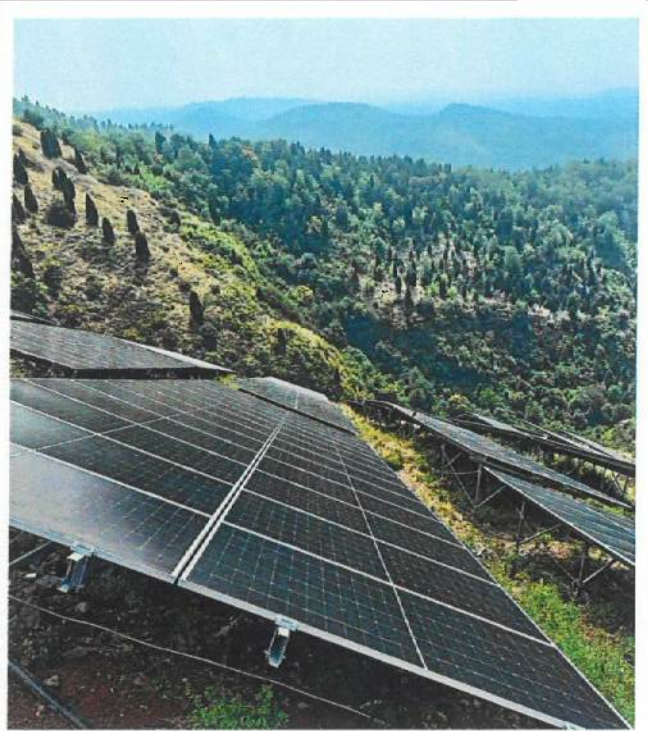
整组组件安装角度调整
