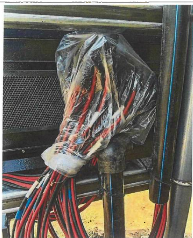
MC 插头保护
