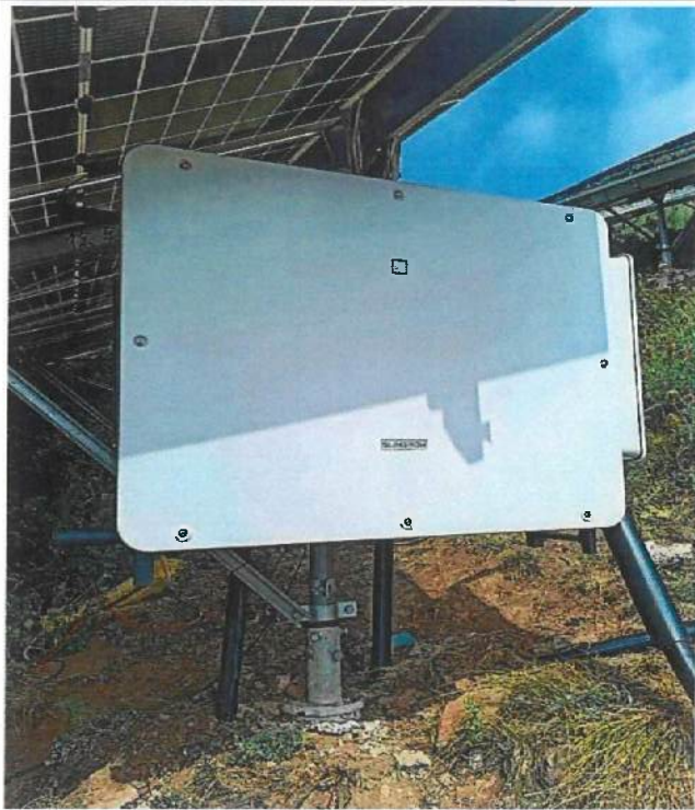
逆变器安装高度调整
