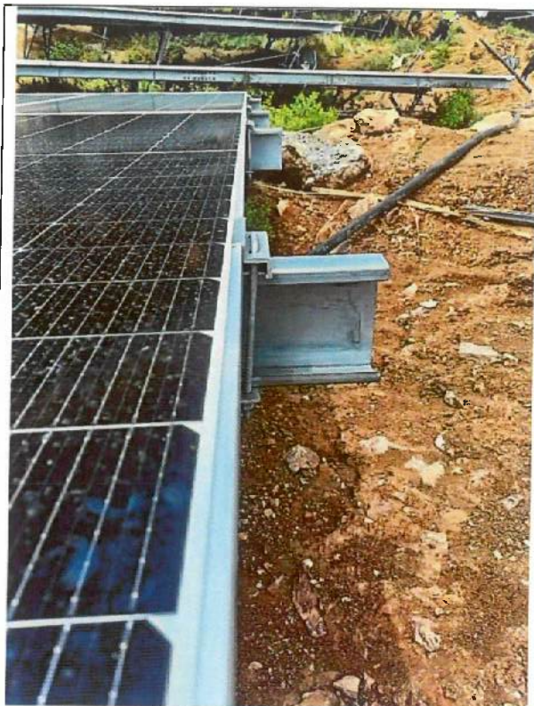
檩条侧边长度预留调整，保证边压受力
