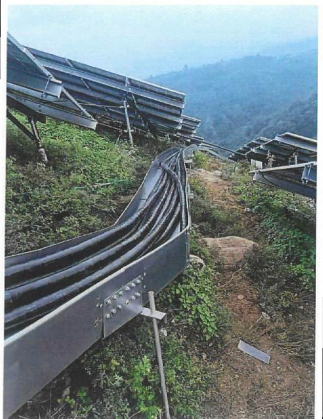
桥架支架调直
