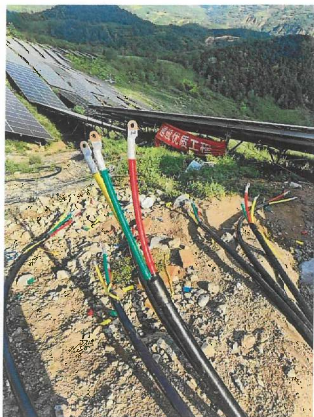
电缆头打磨完成
