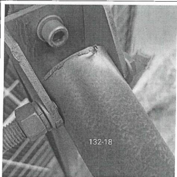
18 连接件生锈已整改
