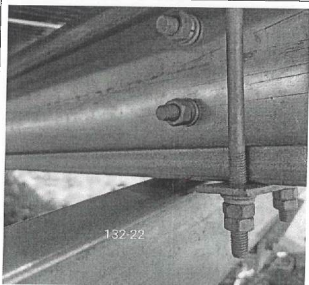
22 檩条悬空已整改
