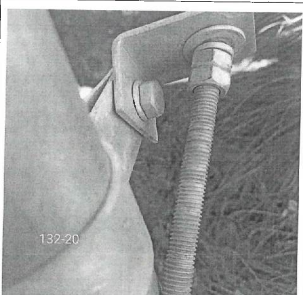
20 背拉杆过长螺丝未紧已整改
