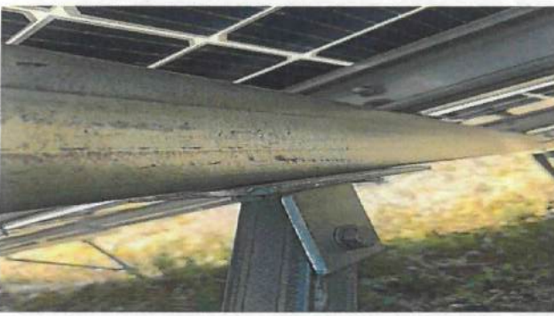
9 连接件拧紧
