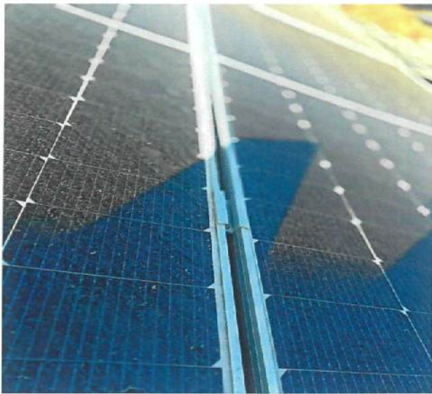
31 压块间隙调整
