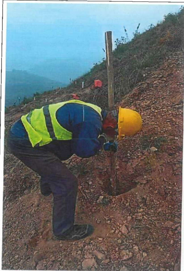
桩基础掏空
