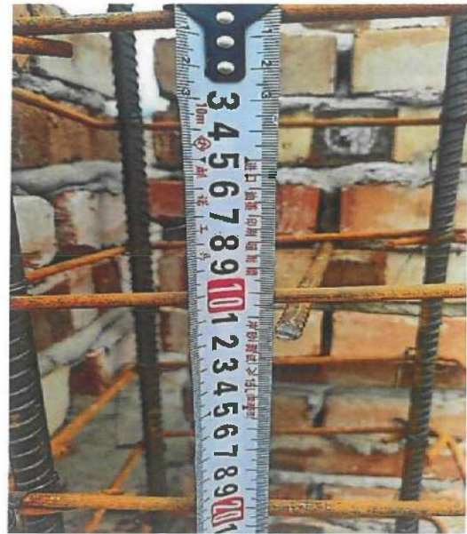
箍筋间距整改
