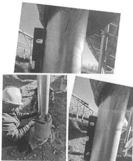
3 立柱角度调整
