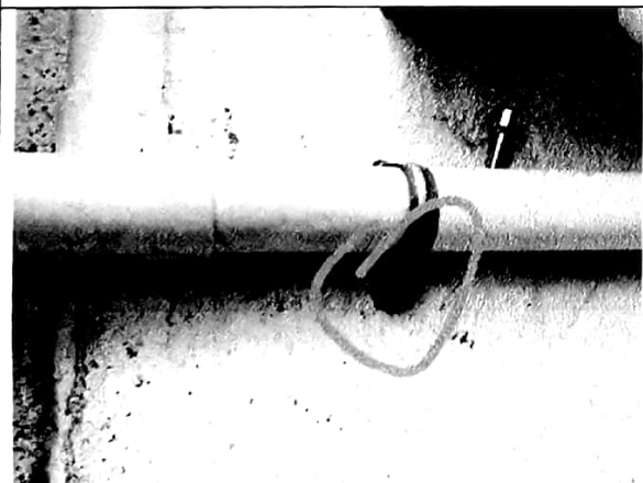
问题 5, 膨胀螺栓未牢固
