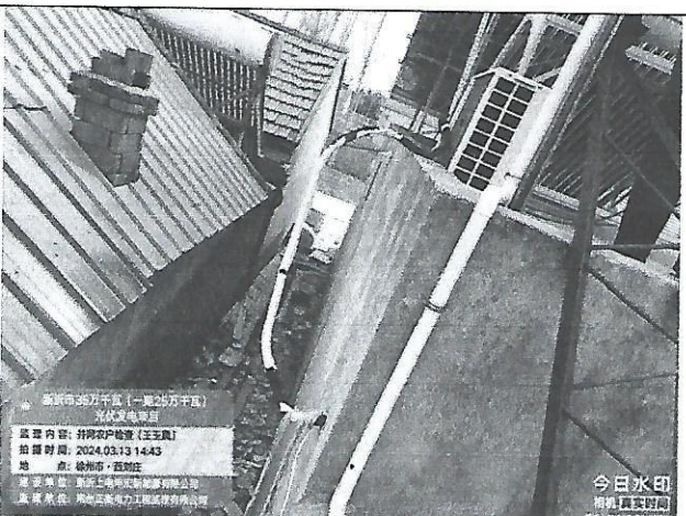
问题 6, 屋面组串接地未连接
