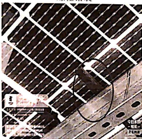
加塞木块，容易造成组件隐裂
