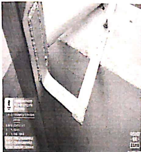
接地扁铁焊接不规范
