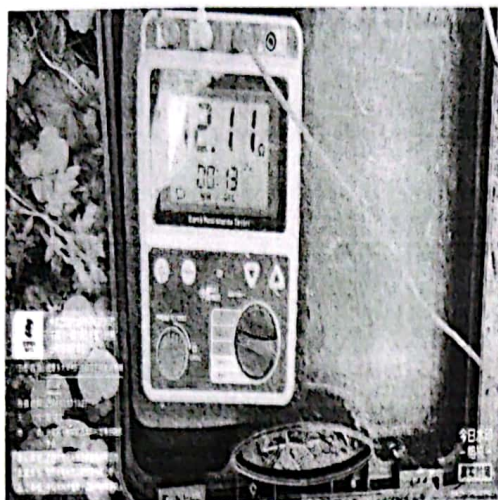
何克彭现场接地电阻检测值
