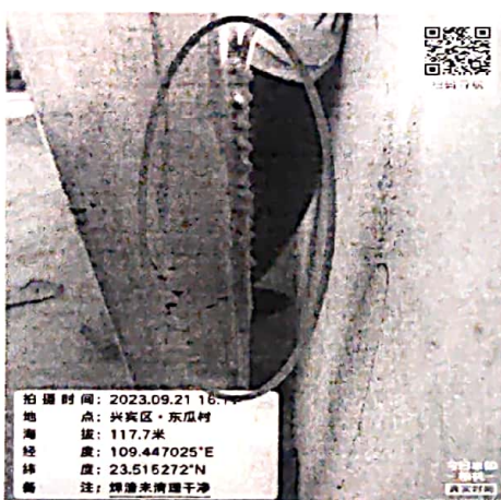
接地扁铁焊接处焊渣未清理
